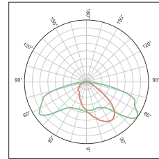
KFLEX4854B ECE M class
