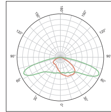
KFLEX3257B ECE M class
