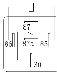
1C 接线图
