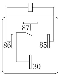
1A 接线图
