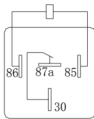
1B 接线图
