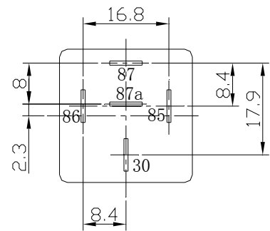
引脚安装图 (快连接式)
