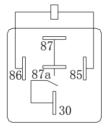
1U 接线图
