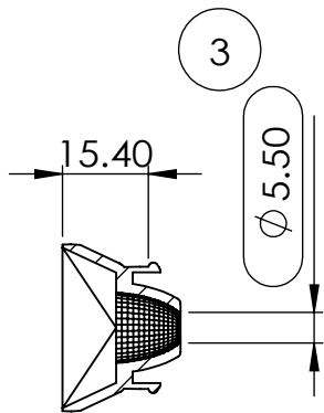
剖面图 A-A
