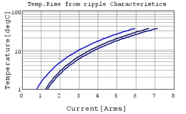
GRM32ER71A476KE15 Temp.rise — 60kHz
