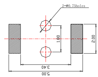
PCB. 焊接图
