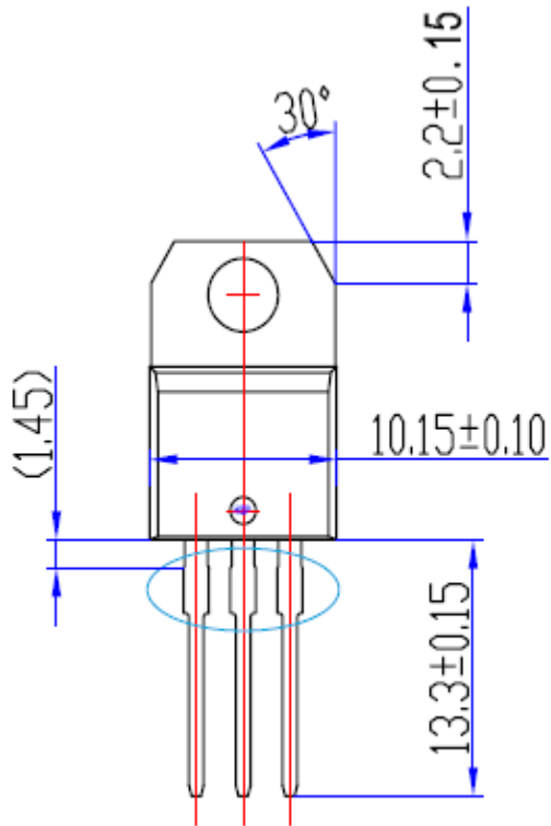
T0-220外形尺寸图:
