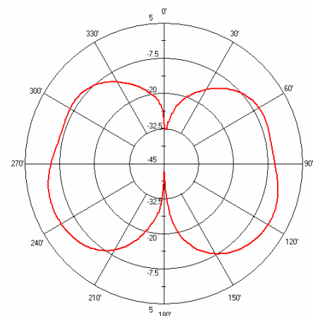
AN9520 E-Plane
