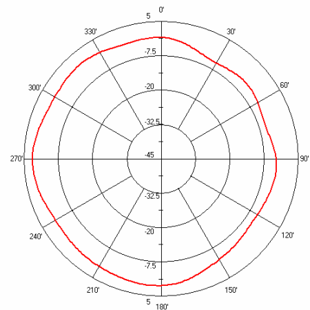
AN9520 E-Plane
