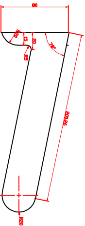
右视图
