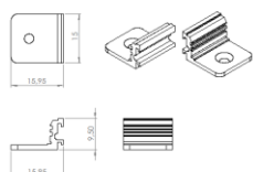
Holder-L
