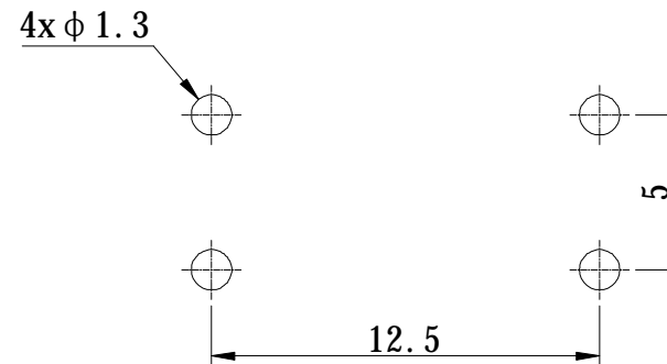
PCB线路板设计参考尺寸 P. C. B. LAYOUT
