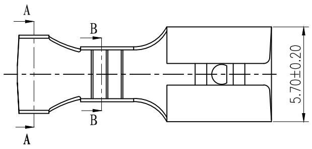
料带图 1:2
