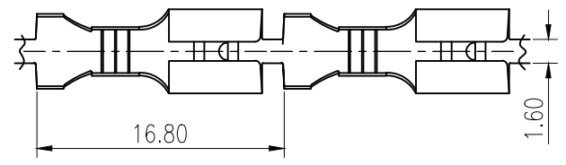
料带图 1:2
